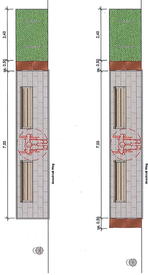
Bankplatz zweifach - Grundrisse M 1:50
