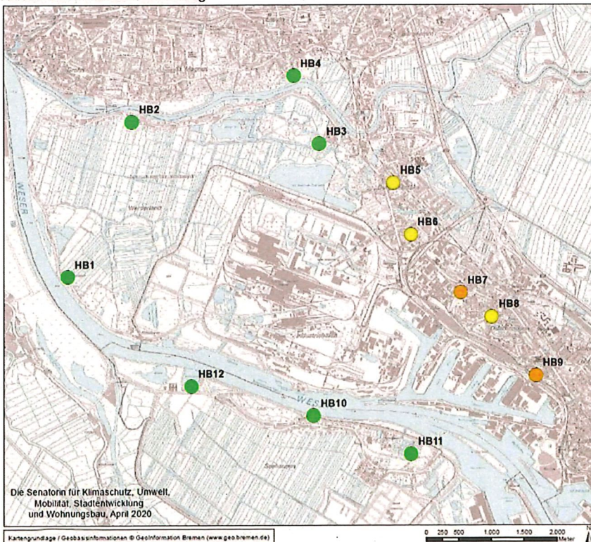
Karte 5 Blei im Staubbiederschlag
