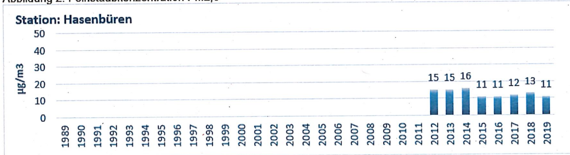
Abbildung 2: Feinstaubkonzentration PM2,5
