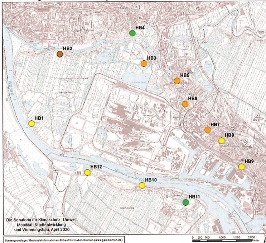
Karte 12 Mangan im Staubbiederschlag
