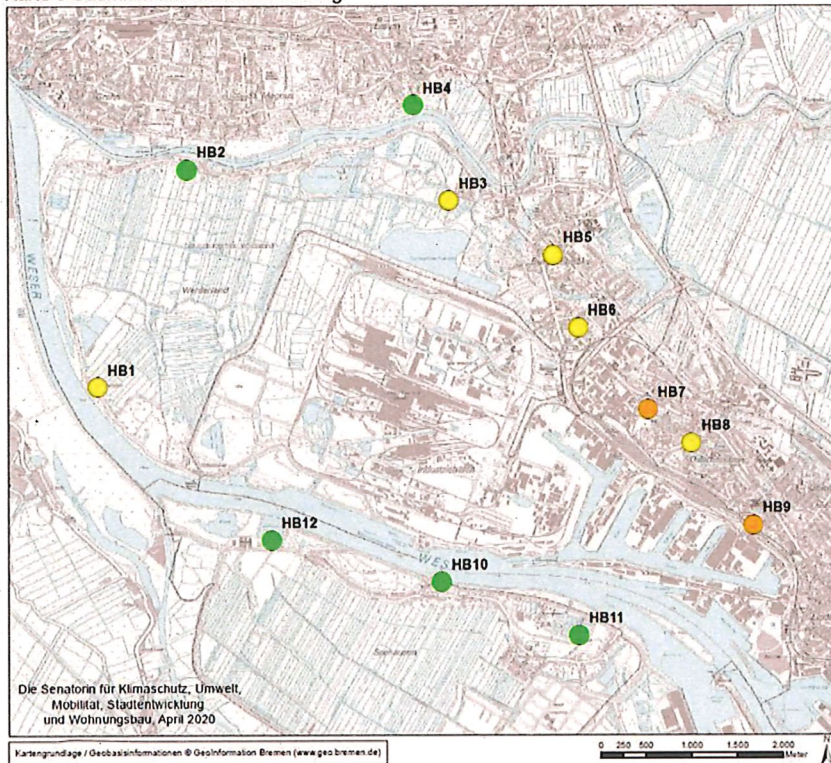
Karte 6 Cadmium im Staubbiederschlag
