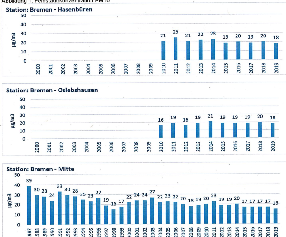
Abbildung 1: Feinstaubkonzentration PM10
