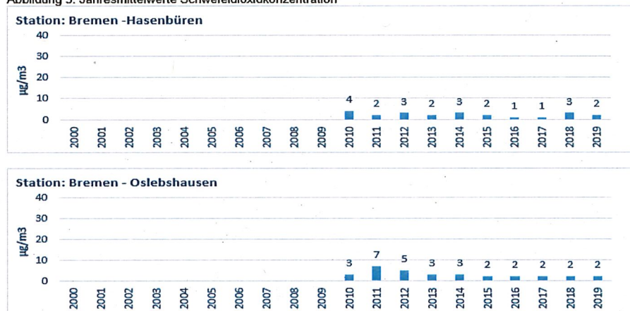
Abbildung 3: Jahresmittelwerte Schwefeldioxidkonzentration
