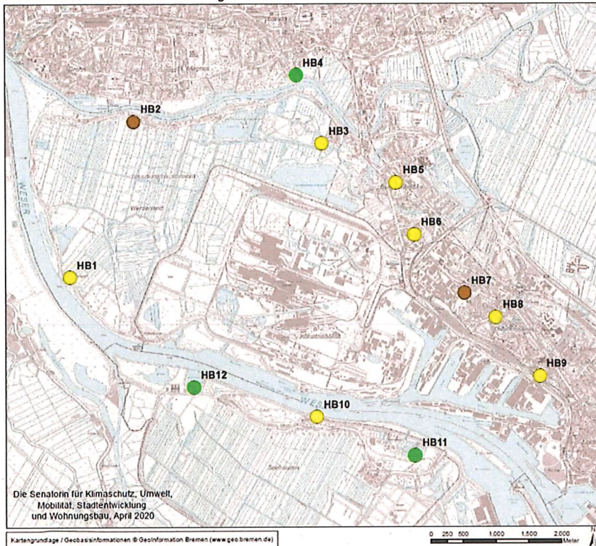
Karte 8 Chrom im Staubniederschlag
