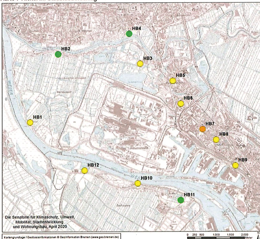
Karte 7 Nickel im Staubbiederschlag
