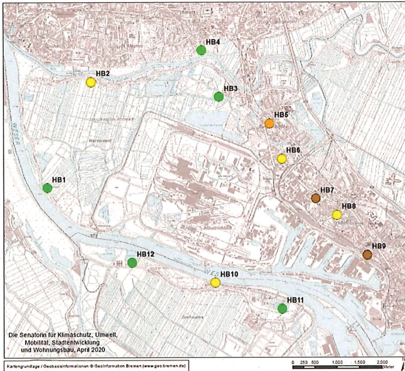
Karte 4 Arsen im Staubbiederschlag
