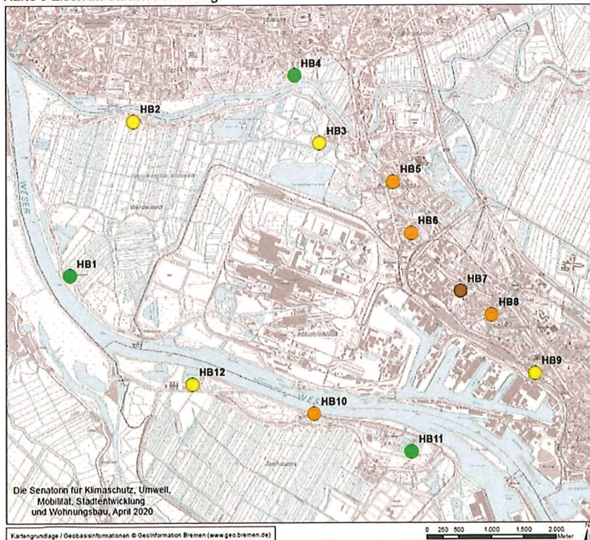
Karte 9 Eisen im Staubniederschlag
