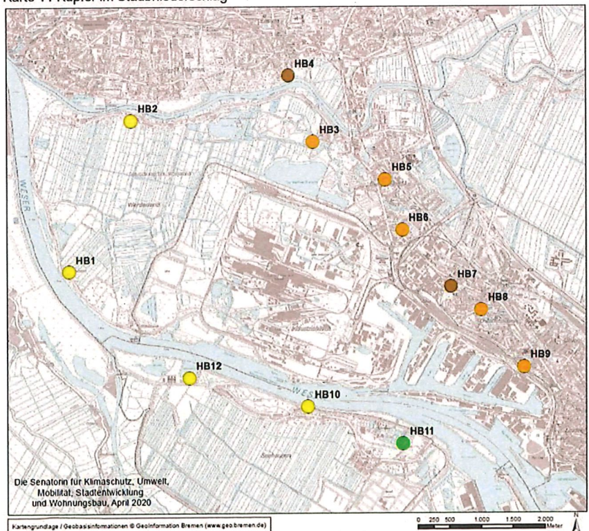
Karte 11 Kupfer im Staubbiederschlag
