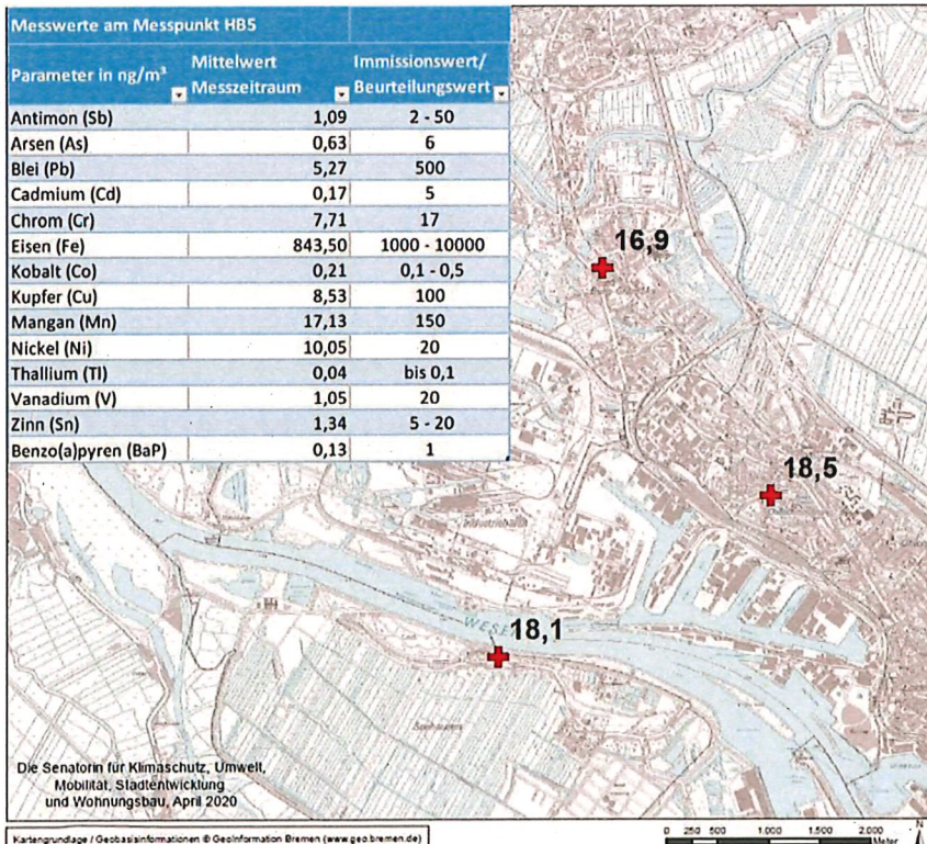
Karte 2 Feinstaub PM10 und Inhaltsstoffe
