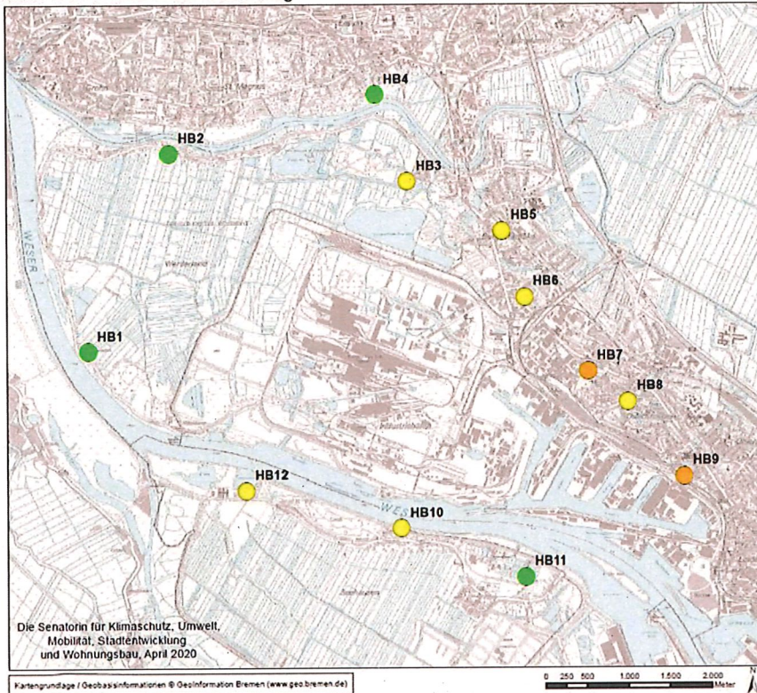
Karte 10 Kobalt im Staubbiederschlag
