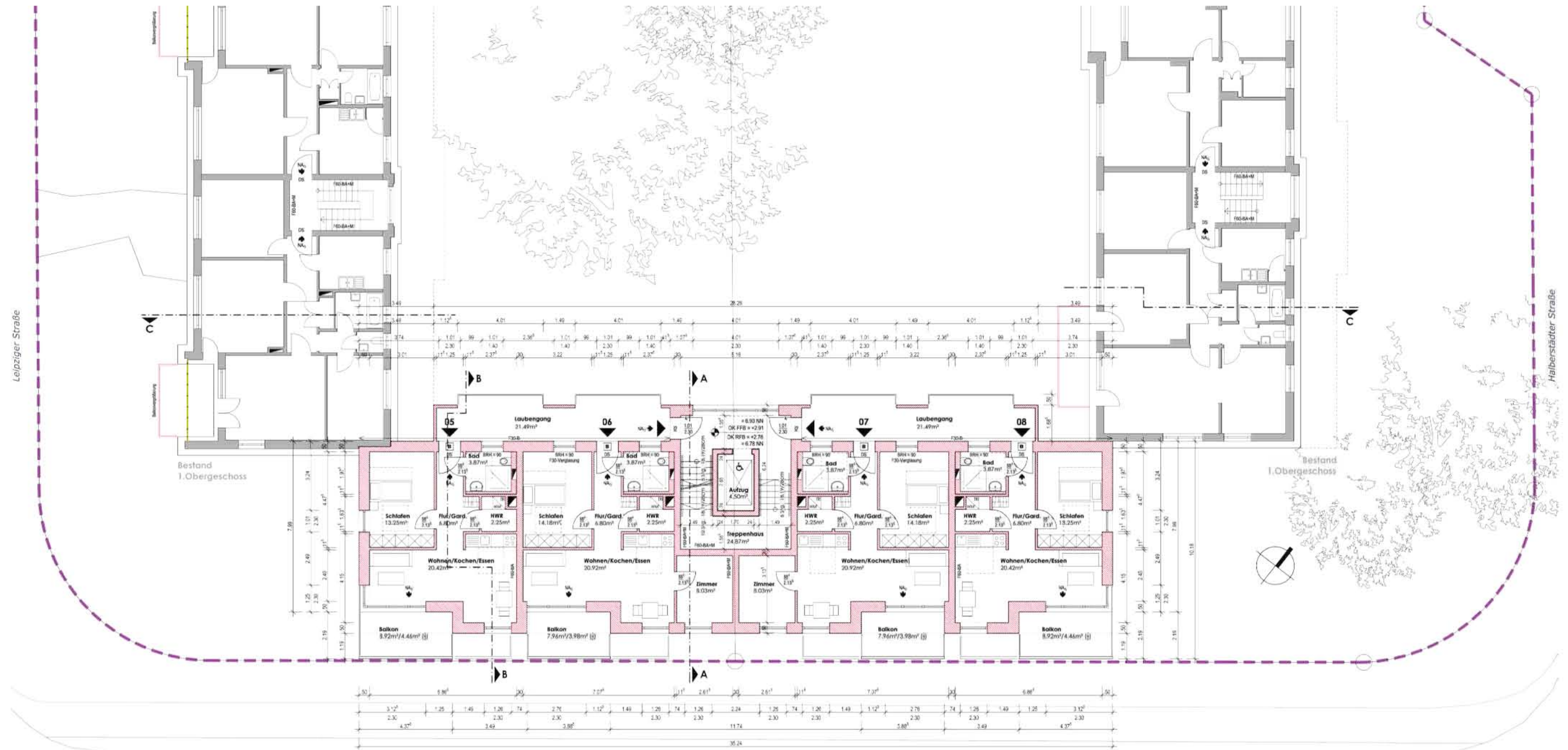
GRUNDRISS 1.OBERGESCHOSS NEUBAU
