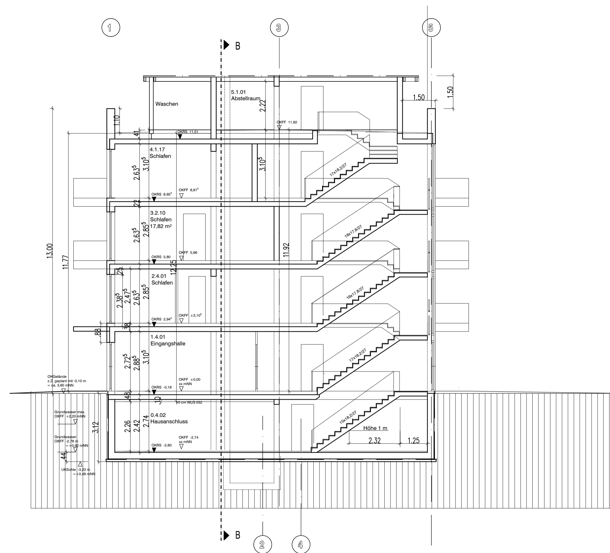
Schnitt A-A
