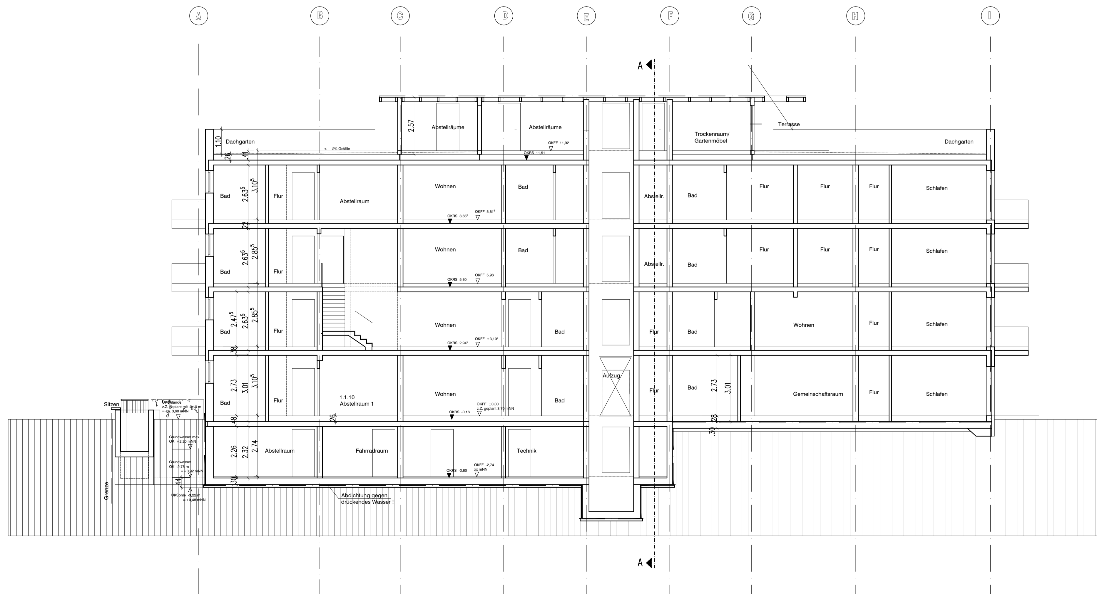
Schnitt B-B
